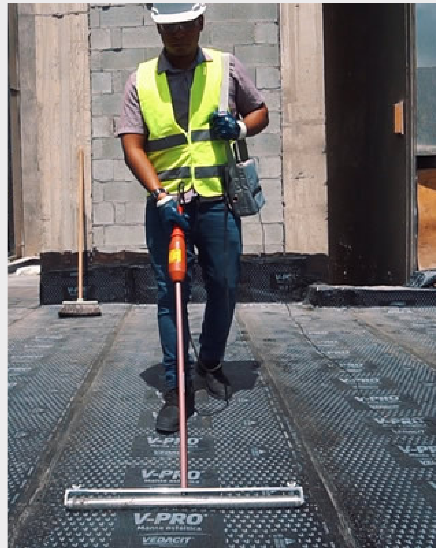
Realização do Teste de Estanqueidade
